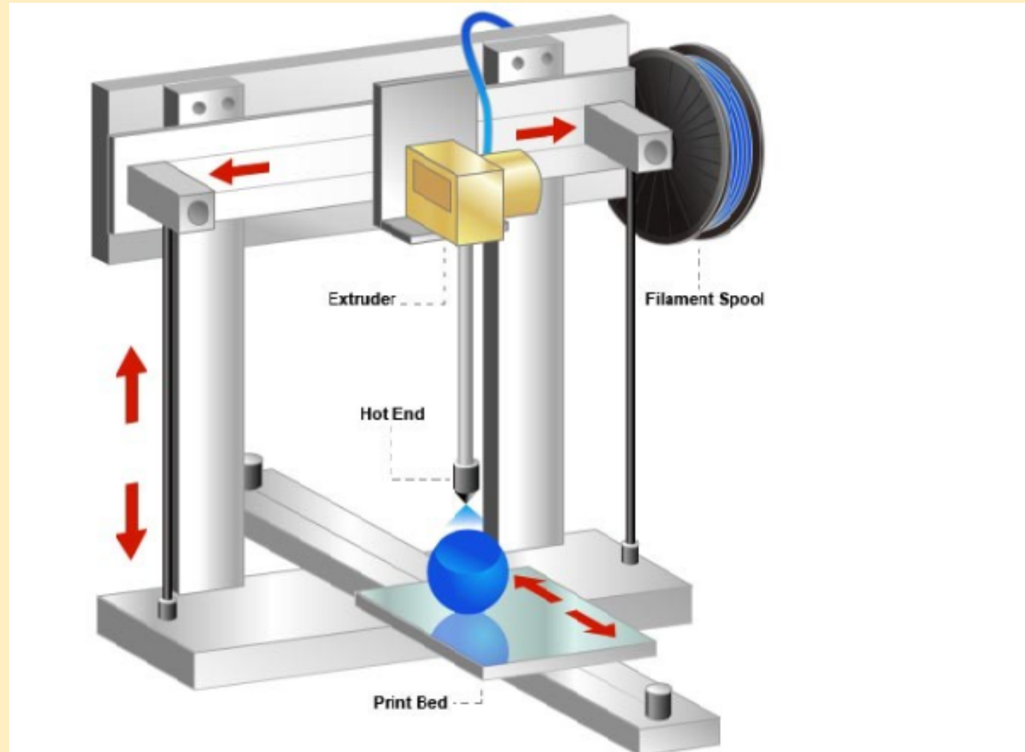
Figure – Schéma d'une imprimante 3D.
