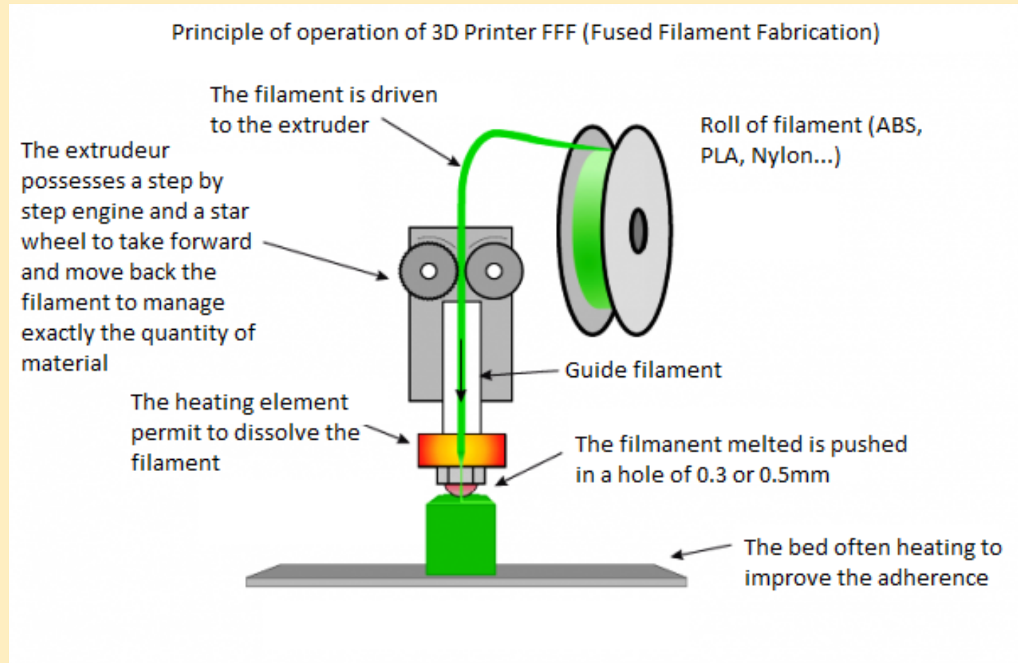
Figure – Schéma d'une tête d'extrusion (extruder).
